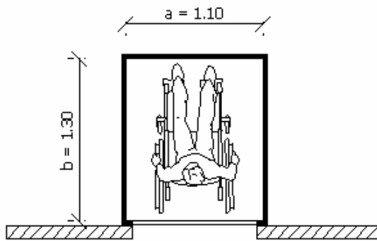
CABINA TIPO 1
